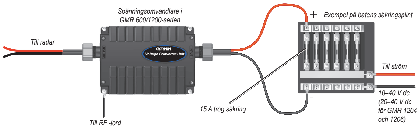
Ansluta spänningsomvandlaren till båtens säkringsplint
