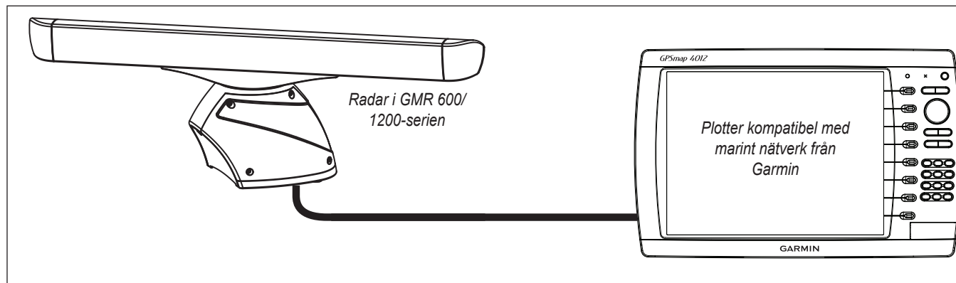
Exempel på fristående marint nätverk från Garmin
