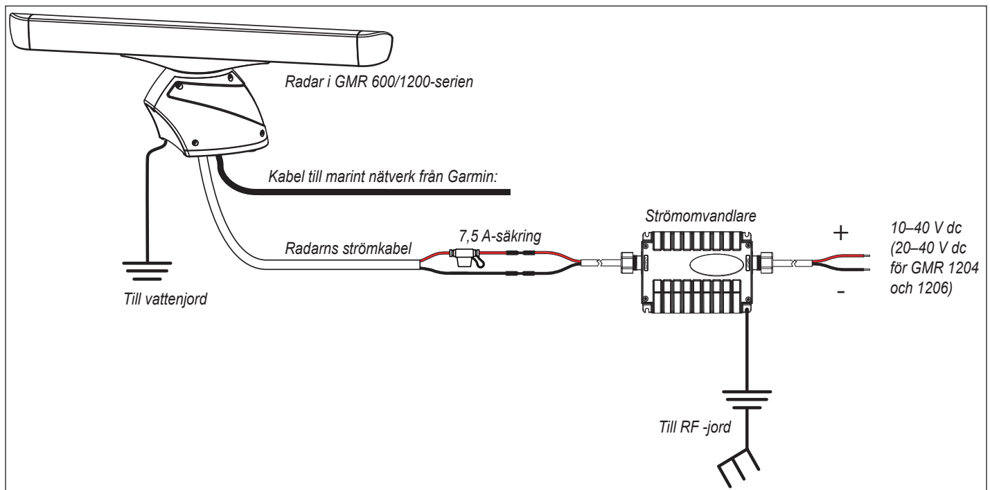
Kopplingsschema
