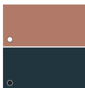
Grafit
